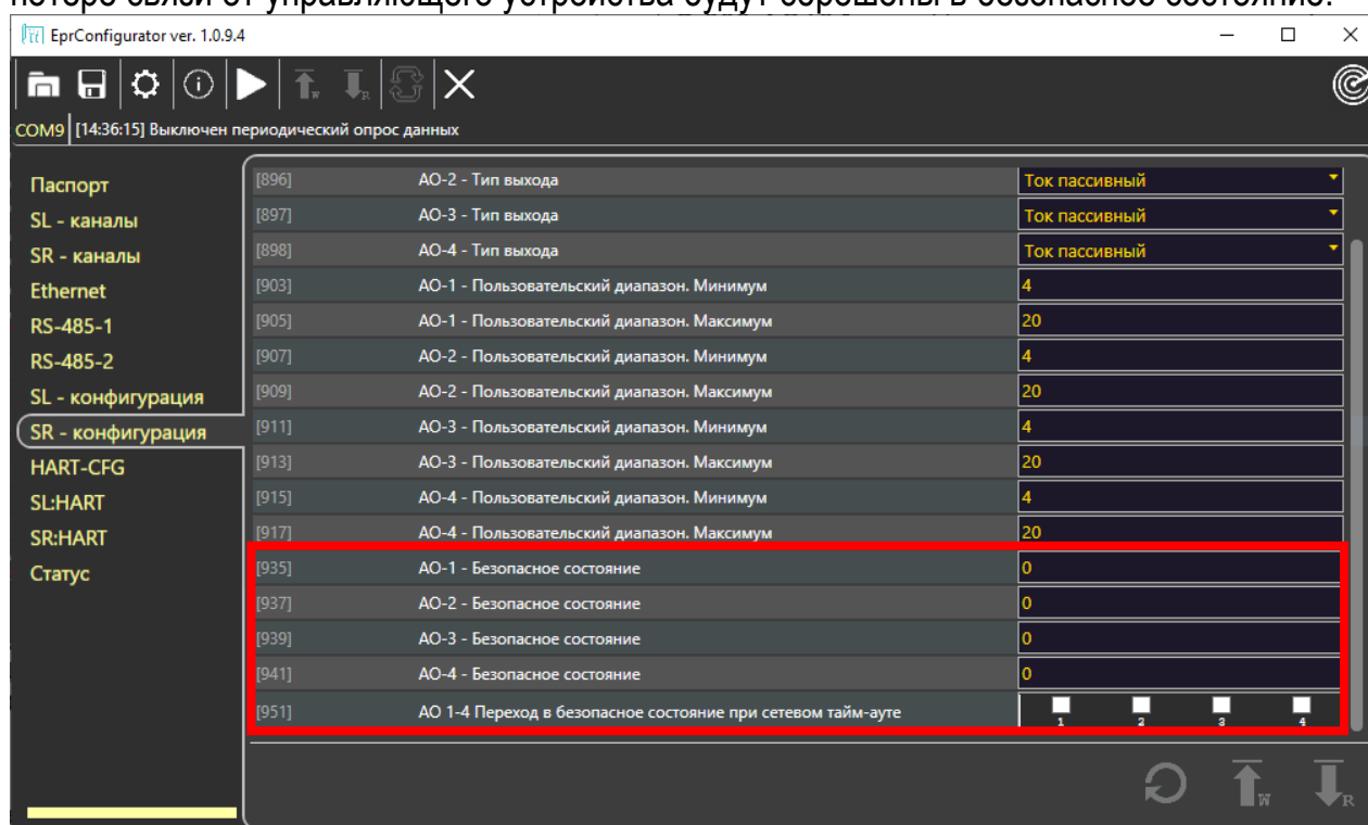
Рисунок 1.6 – Настройка безопасного состояние модуля контроллера Simbol-300 S-300-AO4 HART, S-300-AO8 HART в СПО EprConfigurator
