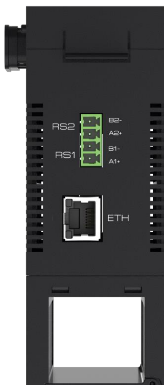
Рисунок 1.3 – Верхняя сторона модуля контроллера Simbol-300 S-300-AO4 HART, S-300-AO8 HART с разъёмами интерфейсов
