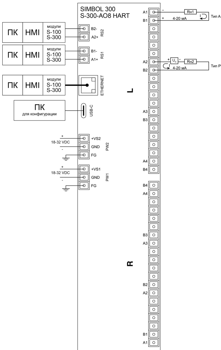
Рисунок 1.5 – Схема подключения модуля контроллера Simbol-300 S-300-AO8 HART (S-300-AO4 HART)
